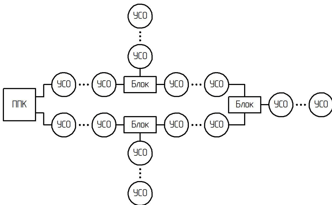
Рисунок 6 - Топология «Смешанная»
