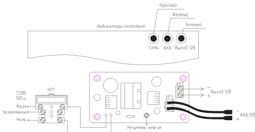
Рисунок 1 Схема подключения Optimus 1230-RM-7
