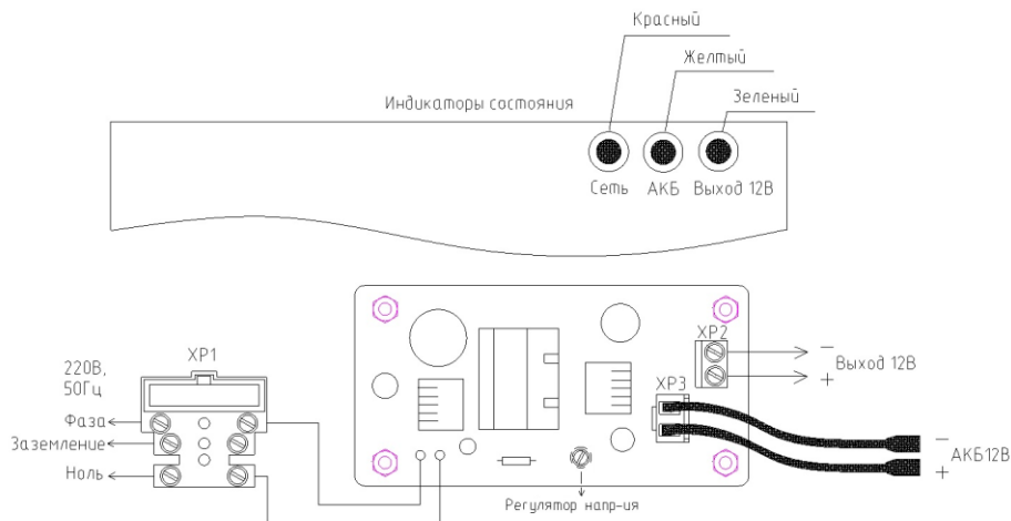
Рисунок 1 Схема подключения Optimus 1230-RM-7
