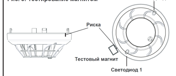
Рис. 3: Тестирование магнитом
