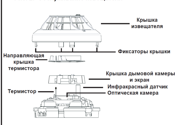
Рис. 2: Обслуживание извещателя
