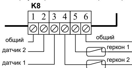
Пример 2. Подключение датчиков и герконов (двухдверный и шлюзовый режимы)
