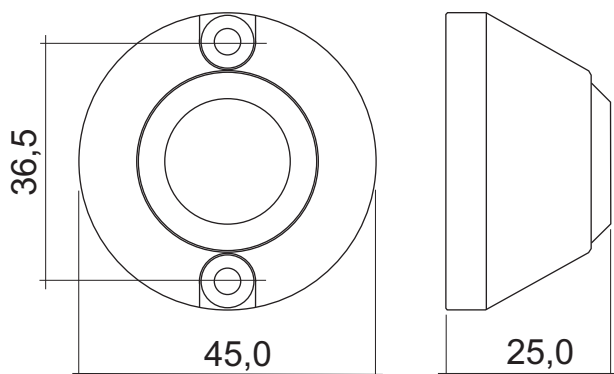
Рис.1 Габариты изделия.
