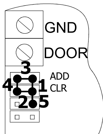
Рис.6 Положения перемычки
