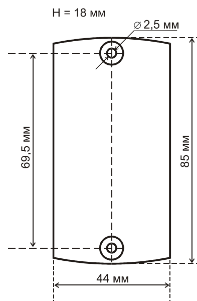
Рис.2 Габаритные размеры
