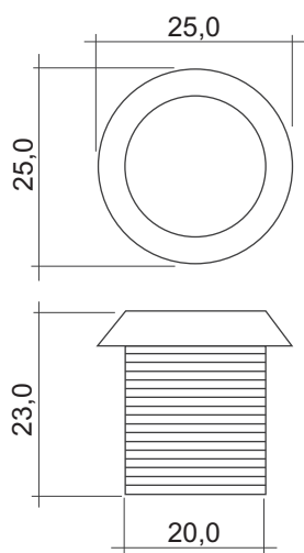
Рис.1 Габариты изделия.
