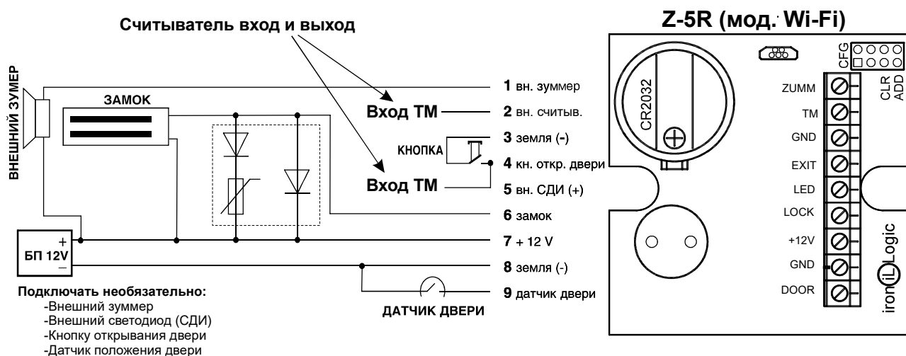
Рис. 3 Схема подключения внешних устройств.
