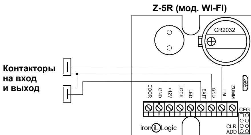
Рис.6 Подключение контакторов.
