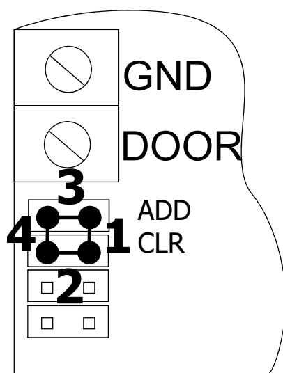
Рис.6 Положения перемычки
