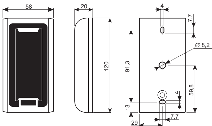
Рис.1 Габариты
