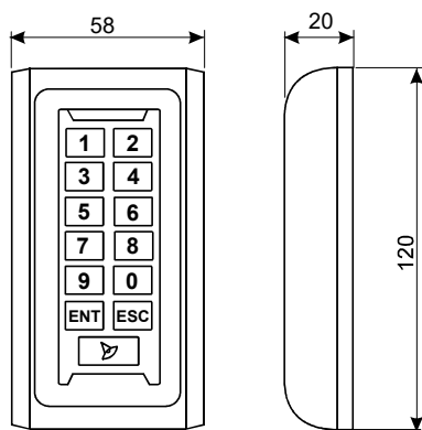
Рис.1 Габариты
