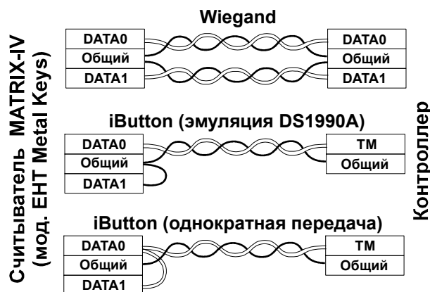
Рис.2 Выбор протокола передачи
