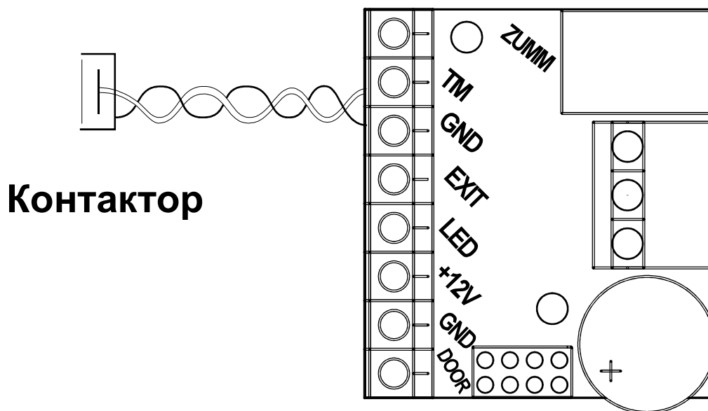
Рис.5 Подключение контактора.
