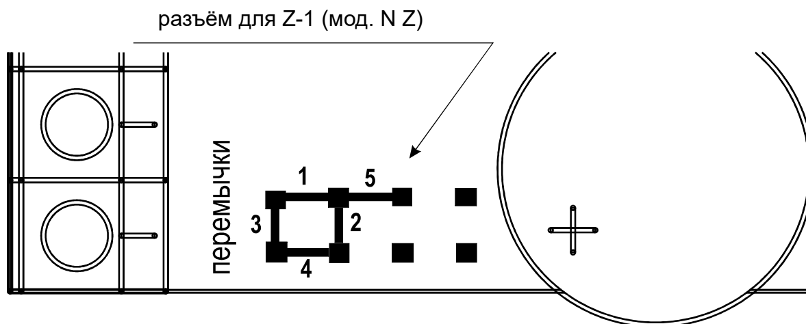
Рис.3 Положение переключателя.
