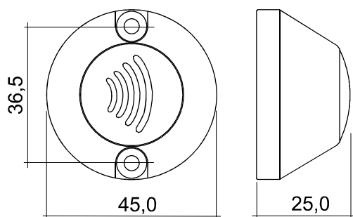
Рис.1 Габариты изделия
