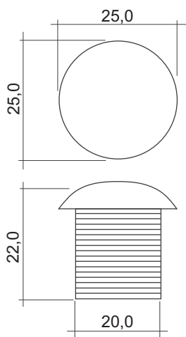
Рис.1 Габариты изделия
