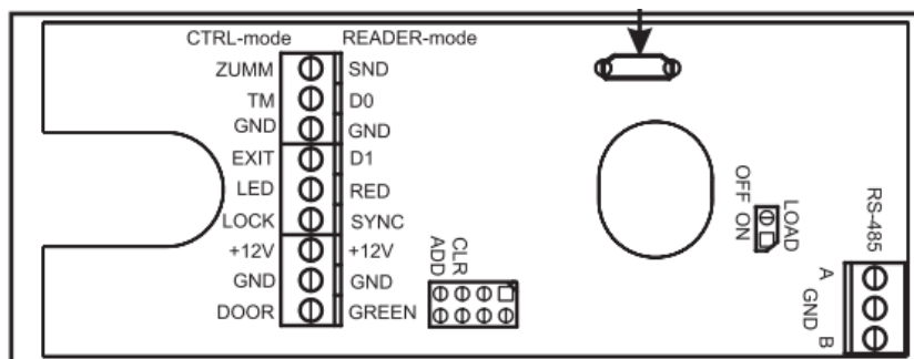
Рис. 1.1 – Клеммы М6.
