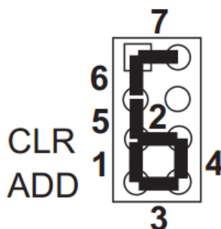
Рис. 1.2 – Переключики М6.
