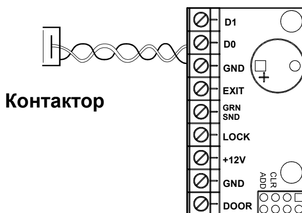
Рис. 4 Подключение контактора
