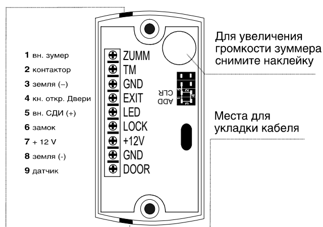
Рис.2 Внешний вид и вид платы контроллера
