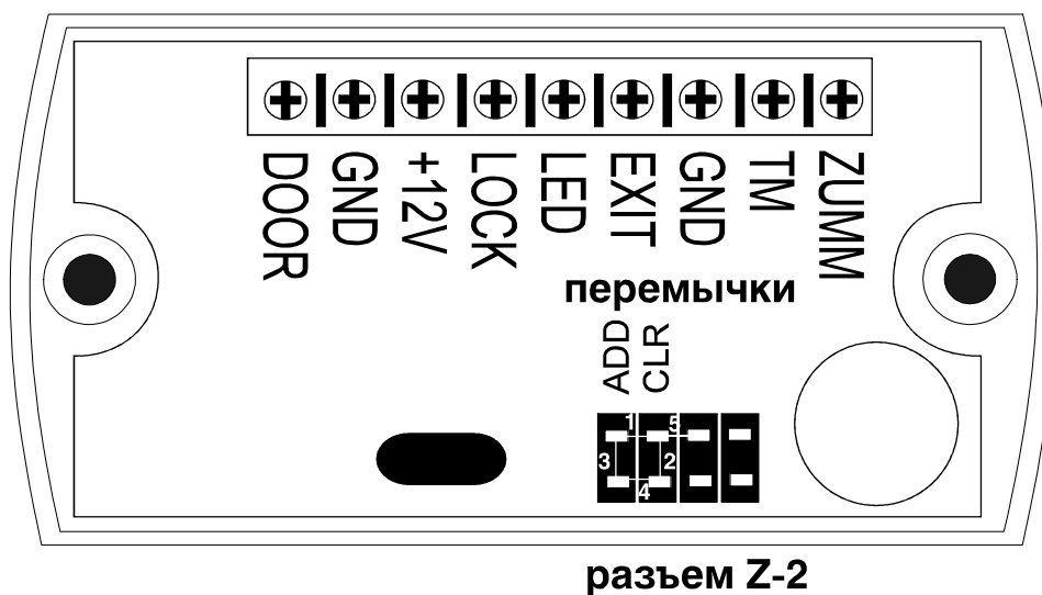
Рис. 3 Положение перемычек
