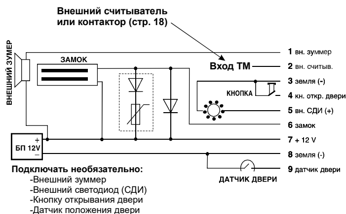
Рис. 6 Подключение внешних устройств
