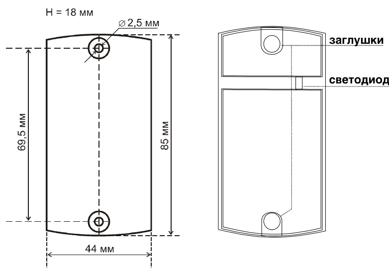
Рис.1 Габаритные размеры контроллера
