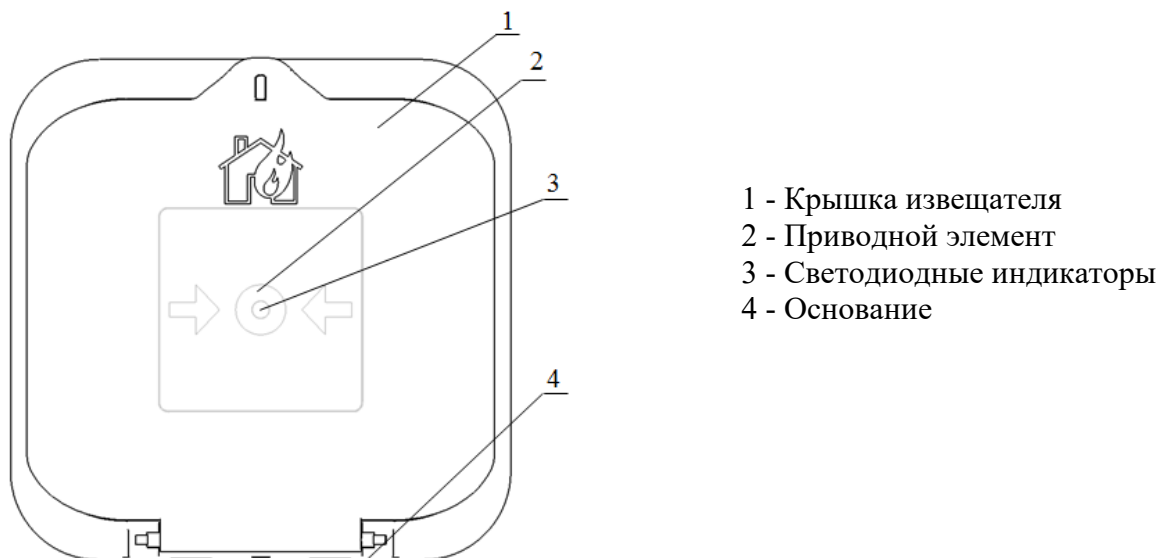
Рисунок 1 - Внешний вид извещателя
