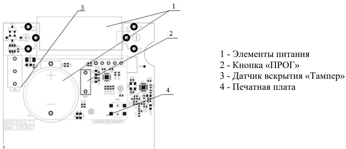
Рисунок 2 - Внутреннее устройство извещателя
