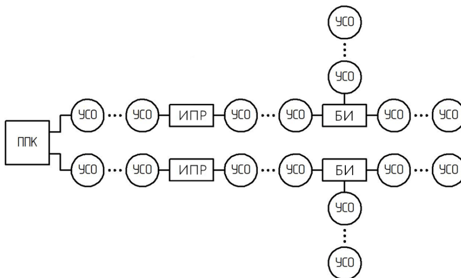
Рисунок 4 - Топология «Дерево»
