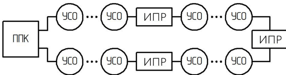
Рисунок 3 - Топология «Кольцо»
