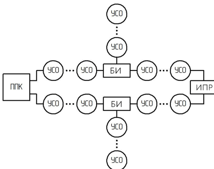
Рисунок 5 - Топология «Смешанная»
