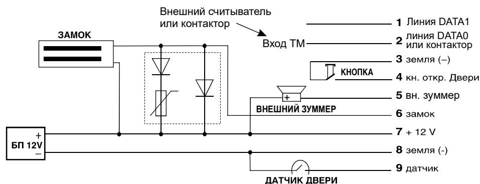
Рис.5 Схема подключения внешних устройств
