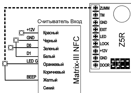
Рис.3 Схема управления внешней индикацией
