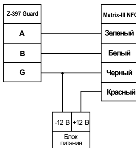
Рис.4 Схема подключения к конвертеру
