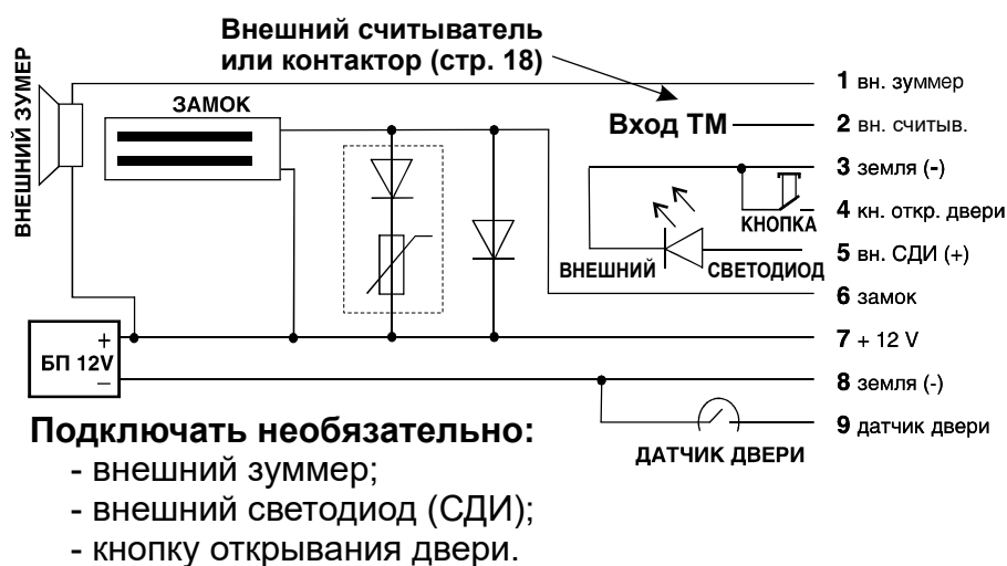
Рис.3 Подключение внешних устройств
