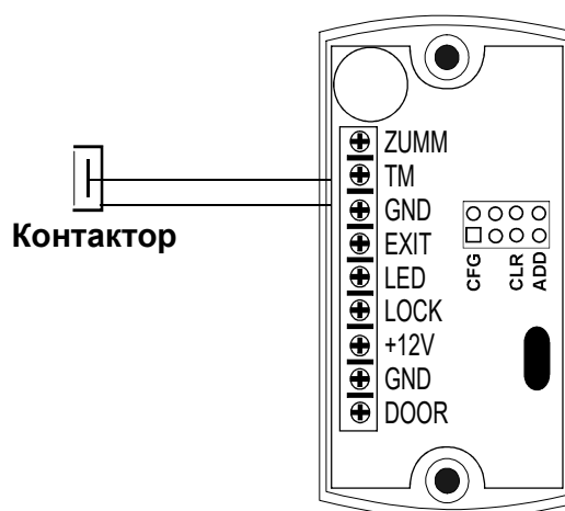
Рис.6 Подключение контактора
