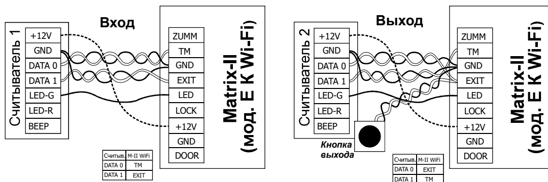
Рис.5 Подключение внешних считывателей по протоколу Wiegand
