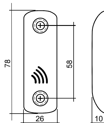
Рис.2 Габариты изделия.
