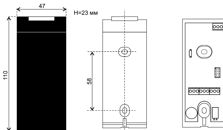
Рис.7 Габариты и монтажные отверстия.
