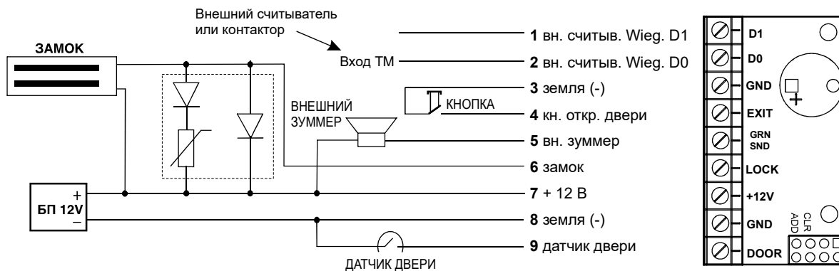
Рис.6 Схема подключения внешних устройств
