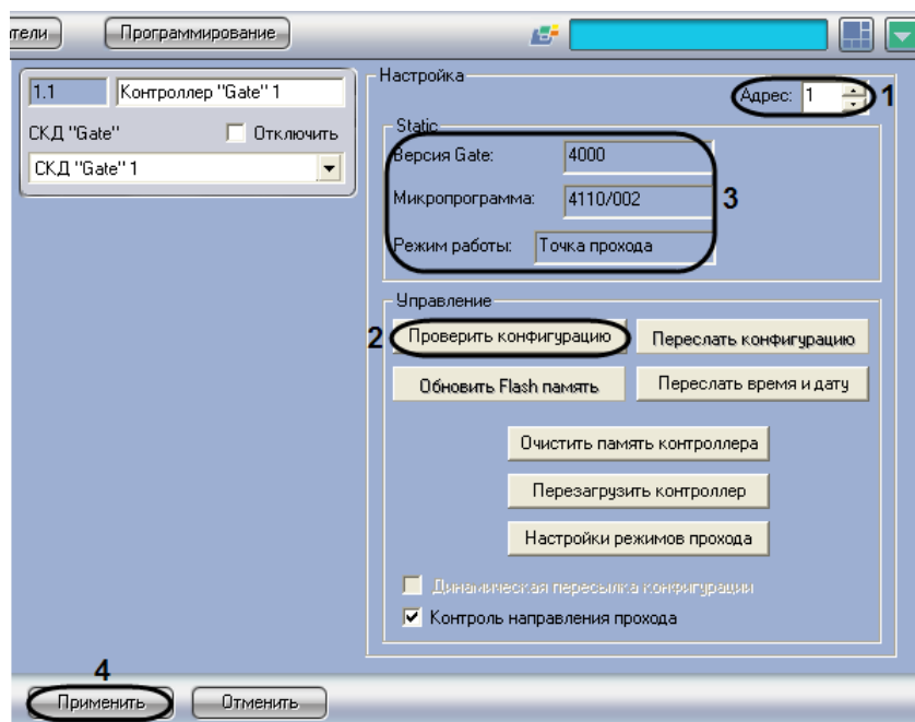
Рис. 3.3-2 Активация контроллера «Gate»
