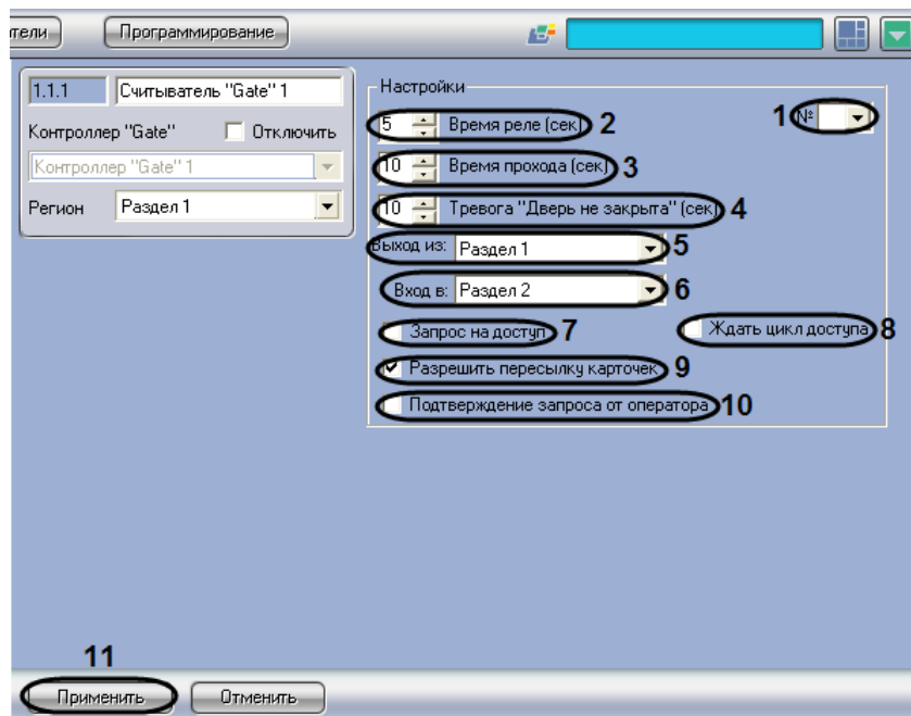
Рис. 3.4-2 Настройка точки доступа СКУД «Gate»
