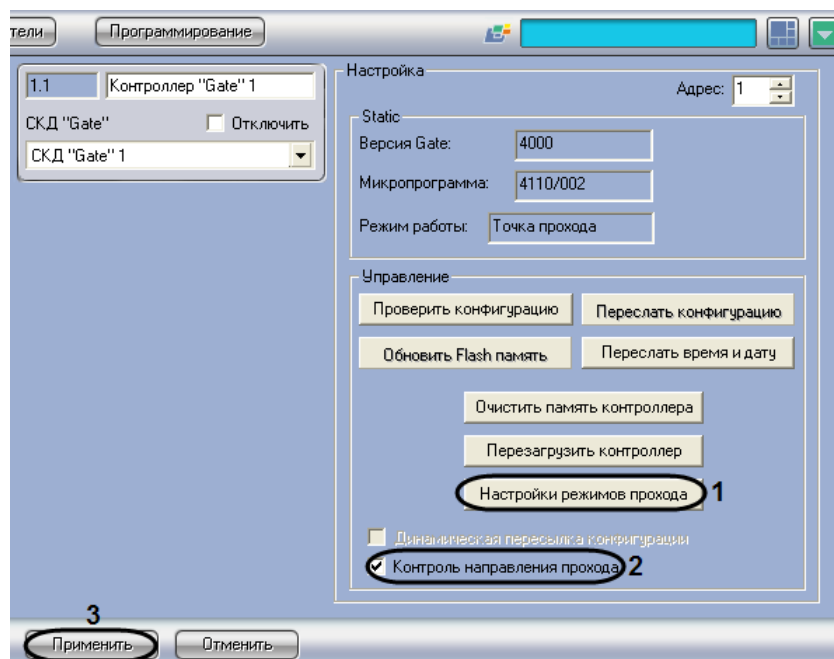
Рис. 3.3-3 Настройка режимов прохода
