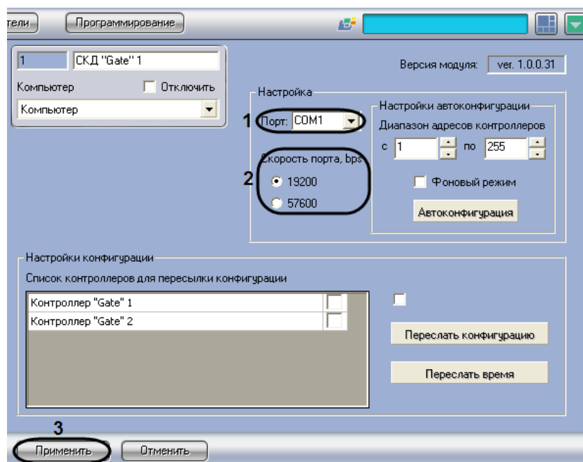
Рис. 3.2-2 Настройка соединения СКУД «Gate» с Сервером «Интеллект»
