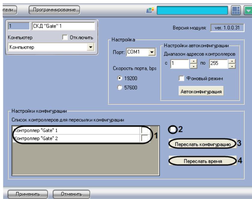
Рис. 3.2-5 Пересылка конфигурации в контроллеры «Gate»
