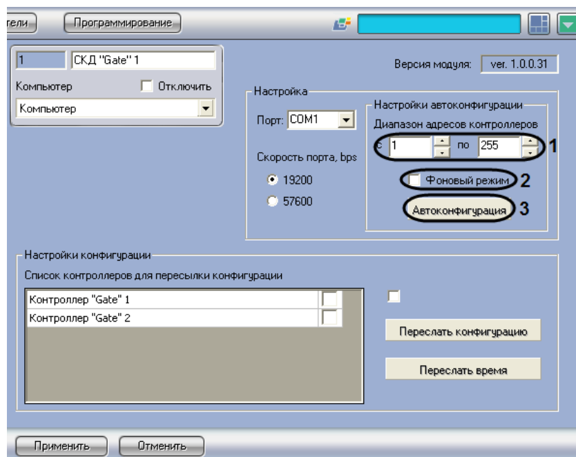
Рис. 3.2-3 Автоконфигурирование дерева объектов модуля «Gate»
