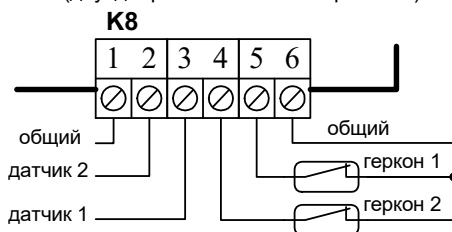
Пример 2. Подключение датчиков и герконов (двухдверный и шлюзовоый режимы)
