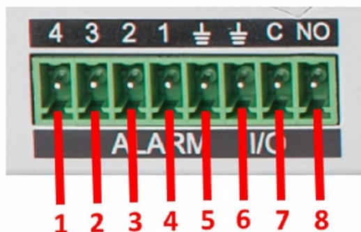
Рис. 1.2.1 Клеммная колодка регистратора
