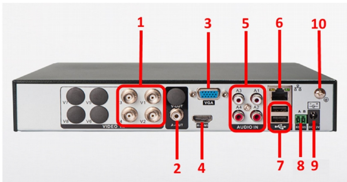
Рис.1.1.1. Задняя панель регистратора (Пример)
