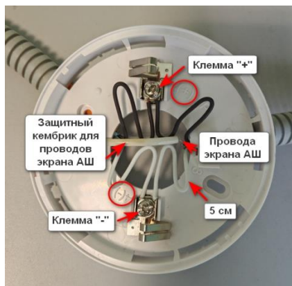
Рис. 3 Подключение и размещение проводов АШ
