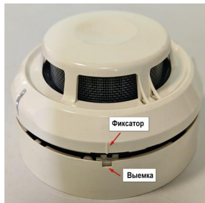
Рис. 4 Монтаж извещателя
