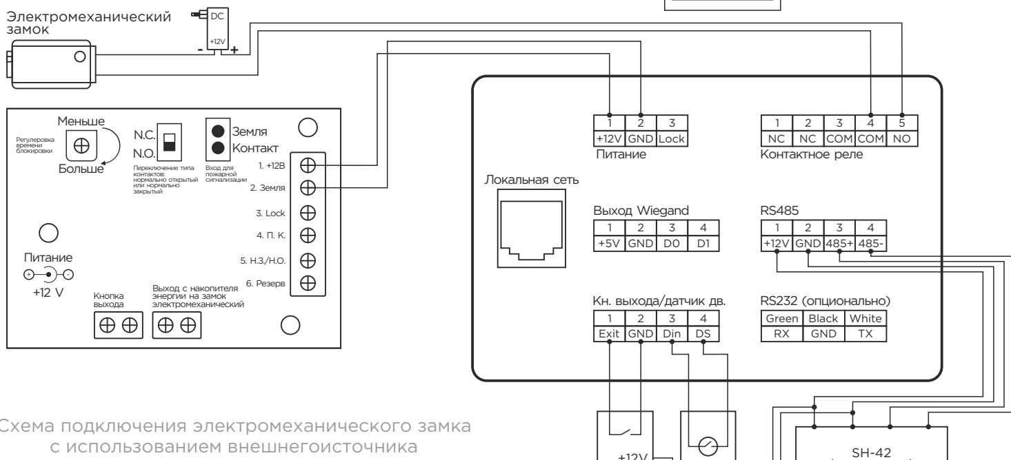
Схема подключения электромеханического замка с использованием блока бесперебойного питания UPS-DP/S
