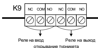
Пример 5. Подключение турникета (турникетный режим)
