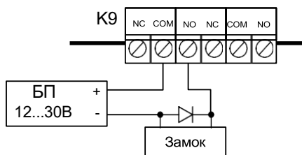
Пример 4. Подключение электромеханического замка (двухдверный и шлюзовой режимы)
