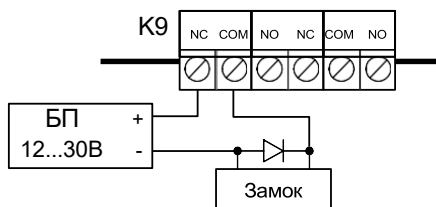
Пример 3. Подключение электромагнитного замка (двухдверный и шлюзовой режимы)
