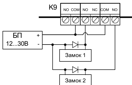
Пример 4. Подключение электромеханического замка (двухдверный и шлюзовой режимы)
