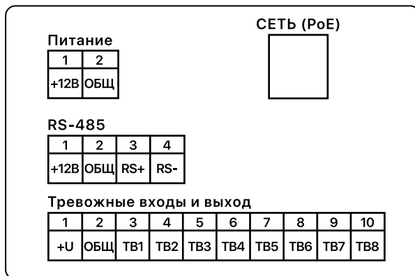
Рис.1 Проводные интерфейсы видеодомофона
