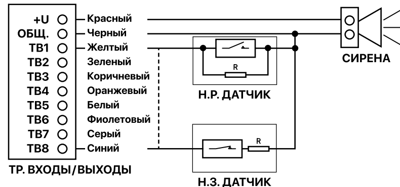
Рис.2 Входы и выход видеодомофона
