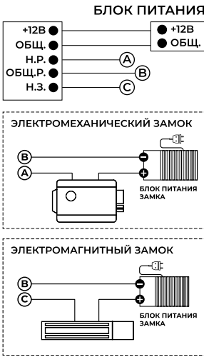
Рис.2 Подключение блока питания и замка
