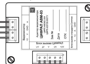
Адаптер видеомонитора с гальваноразвязкой ЦИФРАЛ АВМ-03
