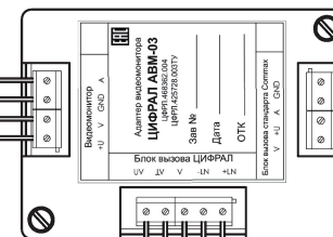
Адаптер видеомонитора с гальваноразвязкой ЦИФРАЛ АВМ-03
