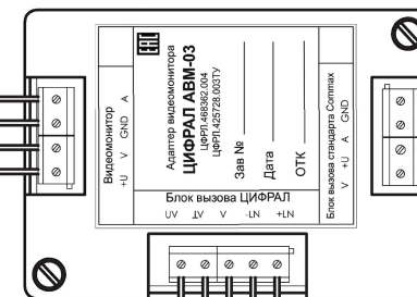
Адаптер видеомонитора с гальваноразвязкой ЦИФРАЛ АВМ-03
