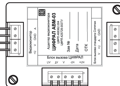
Адаптер видеомонитора с гальваноразвязкой ЦИФРАЛ АВМ-03
