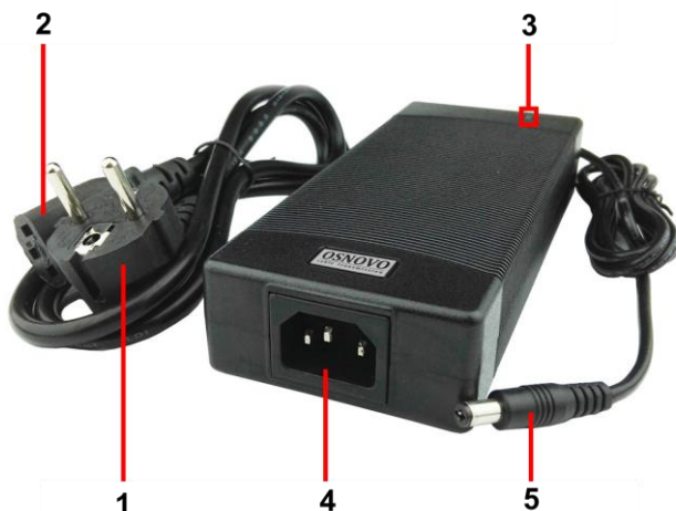
Рис. 2 Блок питания PS-48120, внешний вид, разъемы и индикаторы
