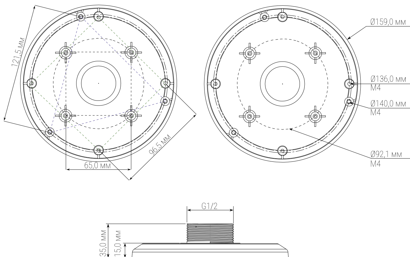
Рисунок 4.1 – Габаритные размеры
