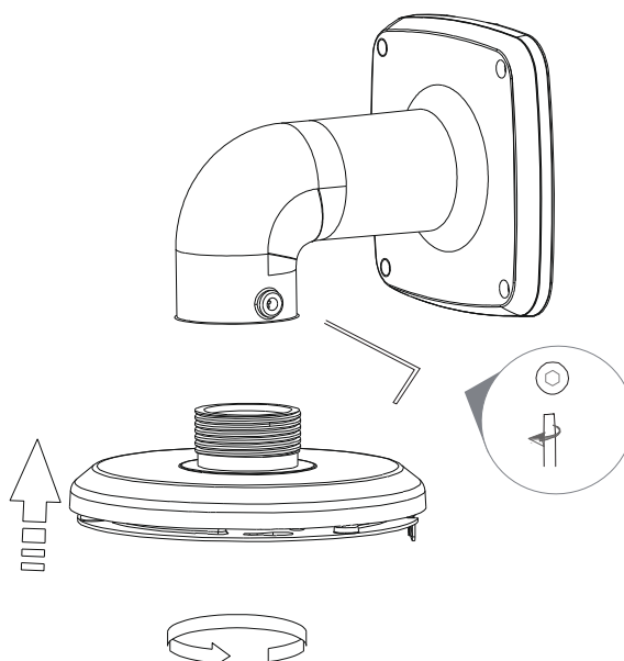
Рисунок 4.4 – Монтаж
