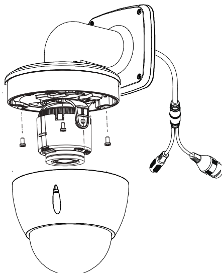
Рисунок 4.5 – Монтаж
