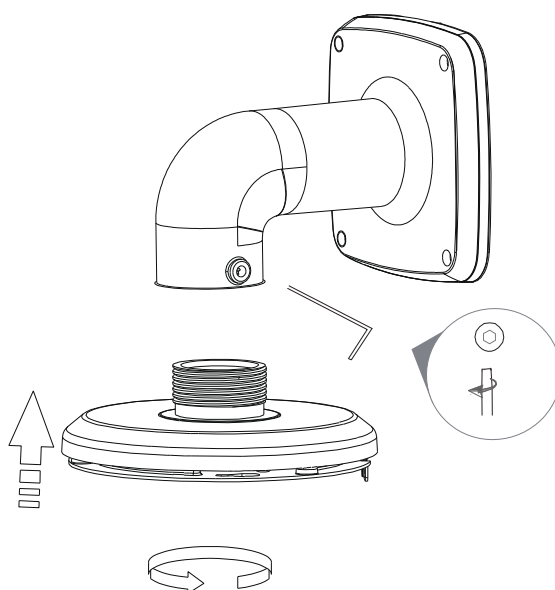
Рисунок 5.5 – Монтаж
