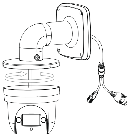
Рисунок 4.6 – Монтаж
