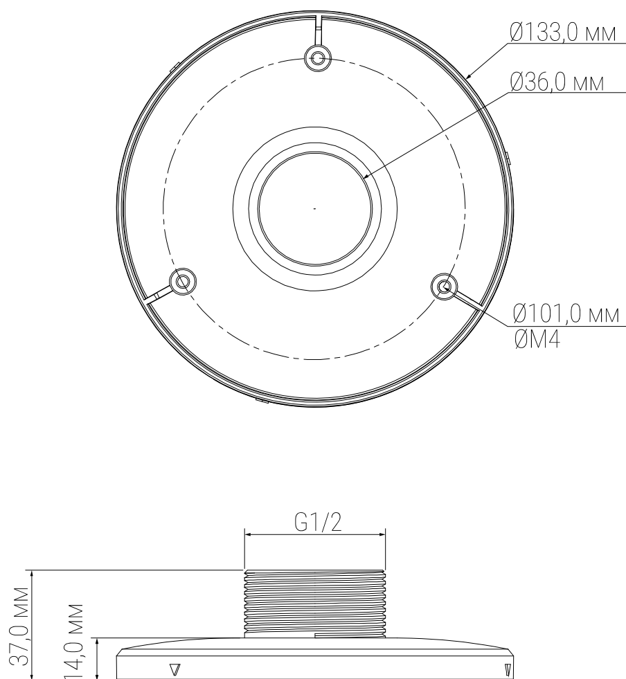
Рисунок 4.1 – Габаритные размеры
