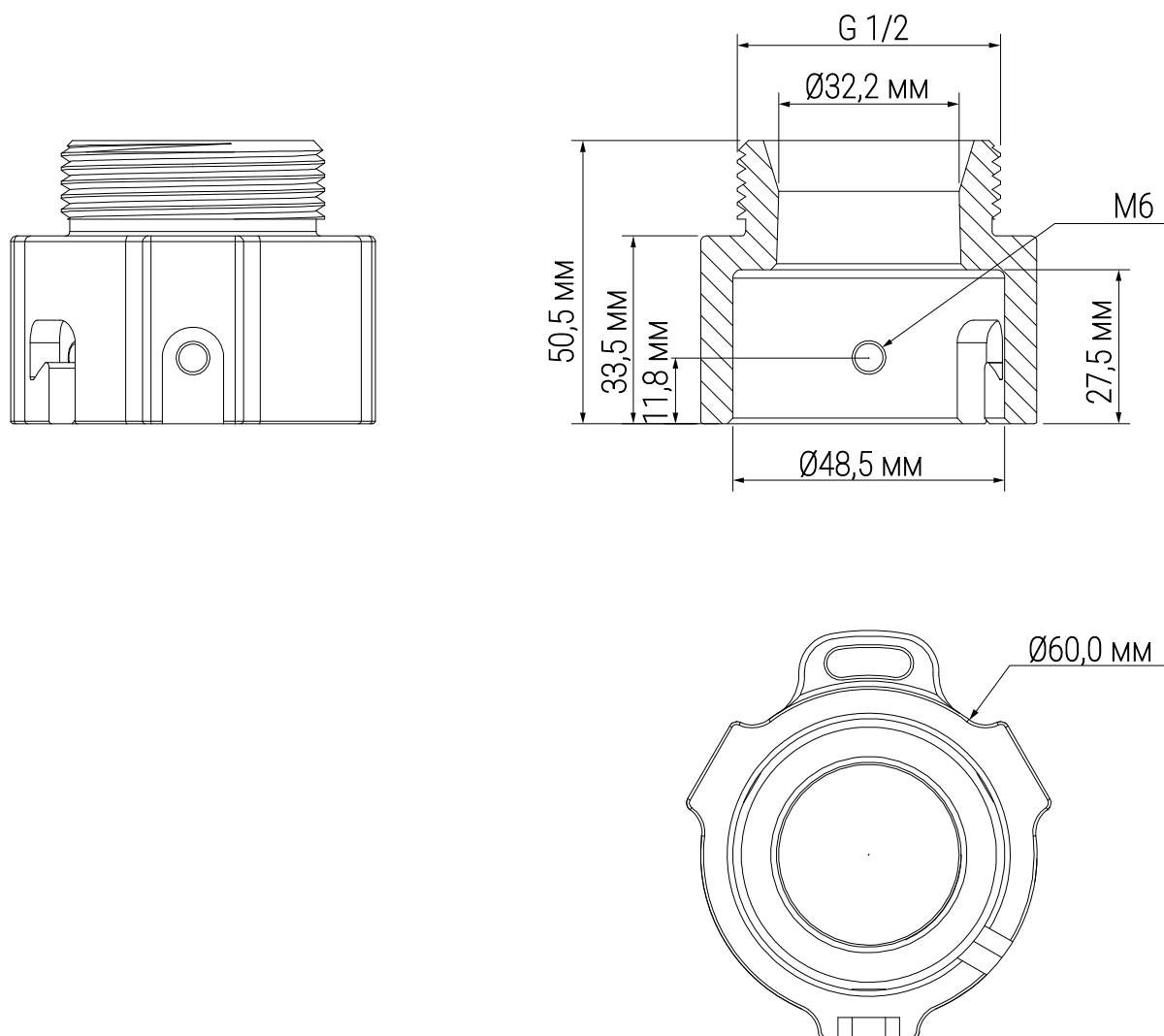
Рисунок 4.1 – Габаритные размеры
