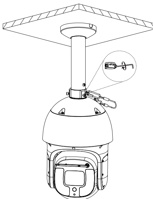
Рисунок 4.7 – Монтаж
