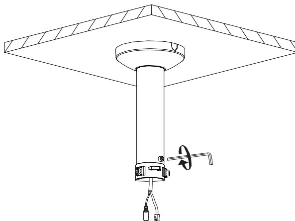
Рисунок 4.6 – Монтаж
