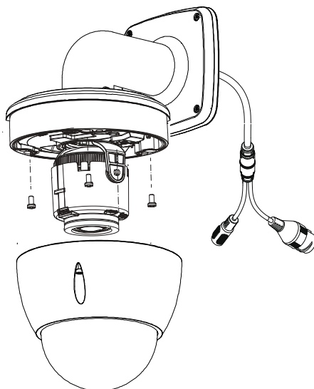
Рисунок 4.5 – Монтаж
