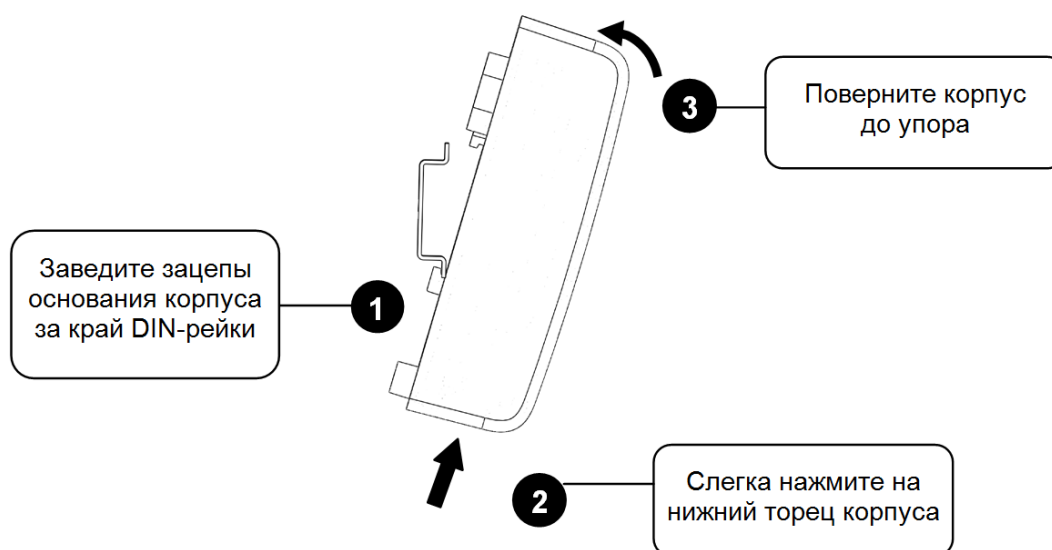
Рисунок 2.2.3.3-1 Монтаж на DIN-рейку C2000P-APP125 апп.1.0
