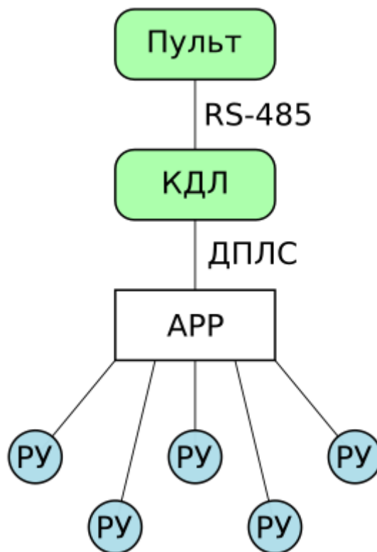
Рисунок 1.1-1 Блок-схема подключения адресных радиоканальных устройств
