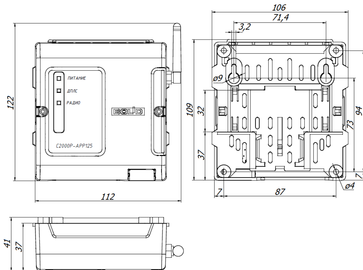
Рисунок 2.2.2.3-2 Габаритные и монтажные размеры C2000P-APP125 апп.14.0
