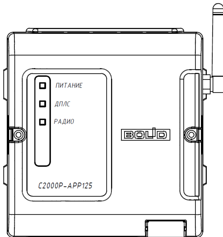
Рисунок 2.2.2.1-2 Внешний вид C2000P-APP125 апп.14.0
