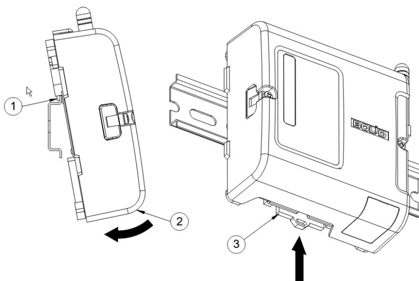
Рисунок 2.2.3.3-1 Монтаж на DIN-рейку C2000P-APP125 апп.1.0
