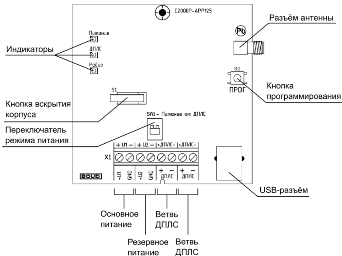
Рисунок 2.2.2.2-2 Расположение элементов на плате апп. 14.0
