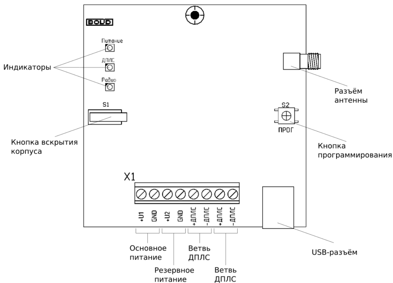
Рисунок 2.2.2.2-1 Расположение элементов на плате апп. 1.0
