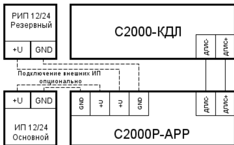
Рисунок 2.2.4-1 Схема подключения радиорасширителя
