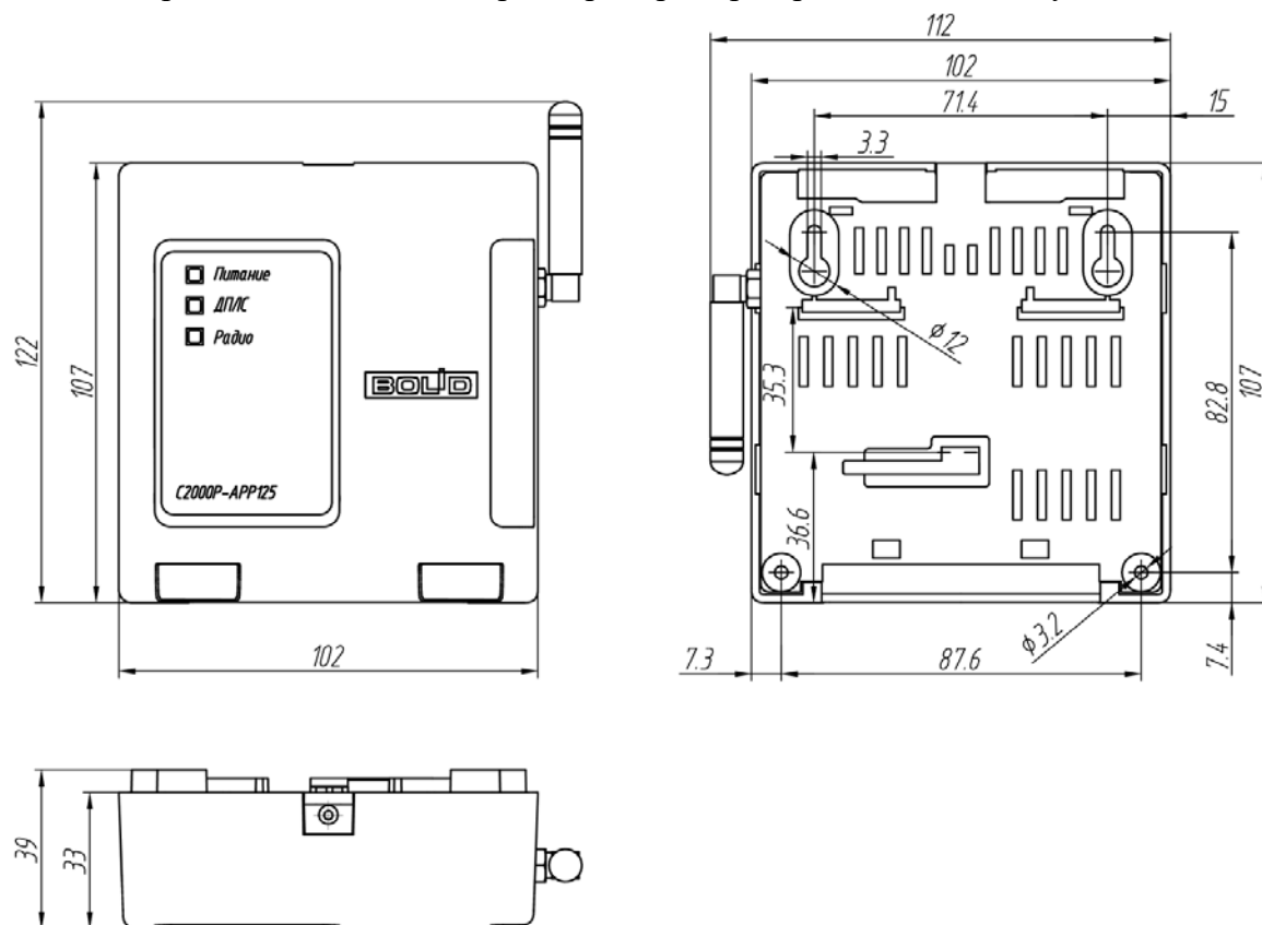
Рисунок 2.2.2.3-1 Габаритные и монтажные размеры C2000P-APP125 апп.1.0
