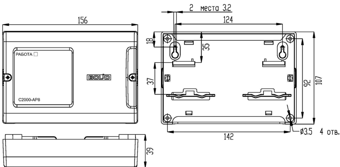
Рисунок 2.2.1 Габаритные и установочные размеры АР8
