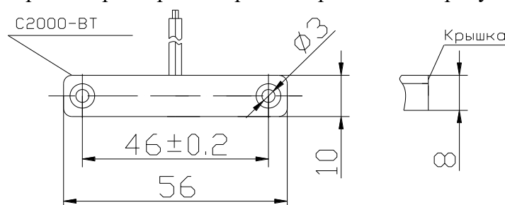
Рисунок 1. Внешний вид и габаритные размеры измерителя
