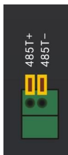
RS485 интерфейс 4 канального регистратора
