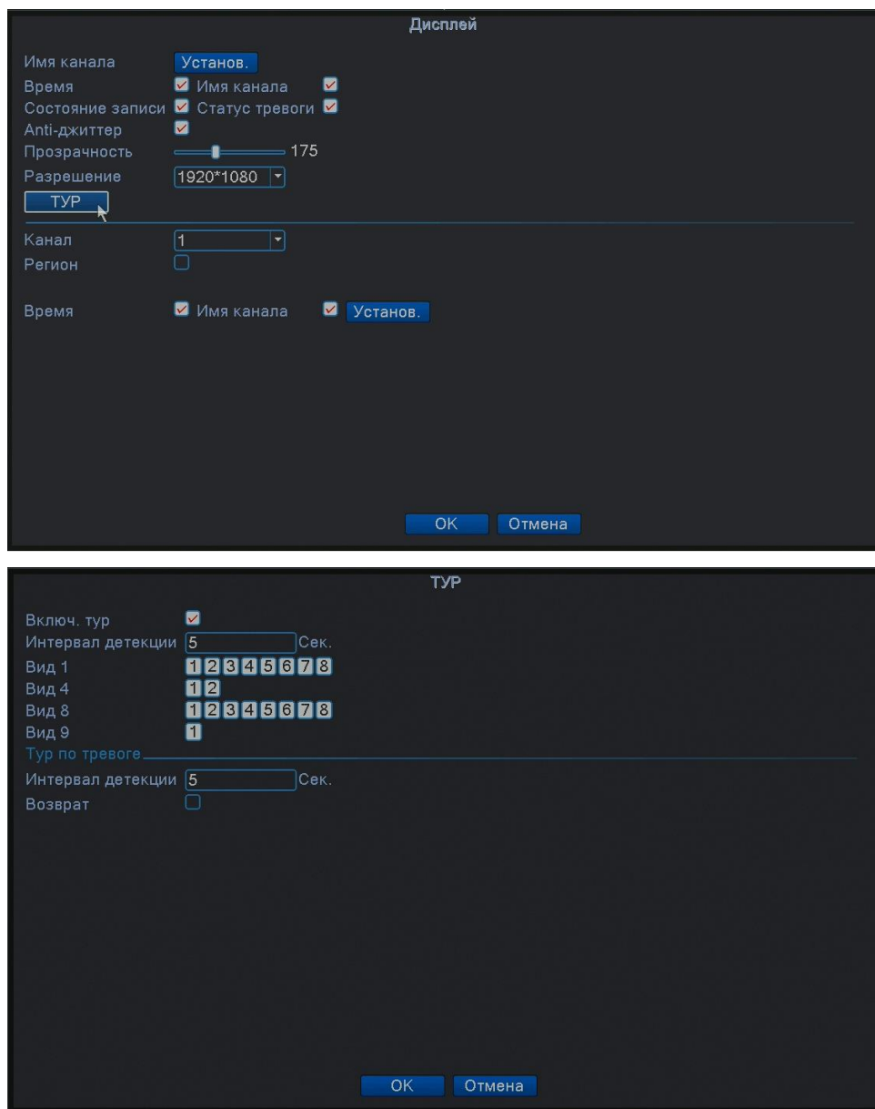
Рисунок 4.39 Настройка тура для дисплея
