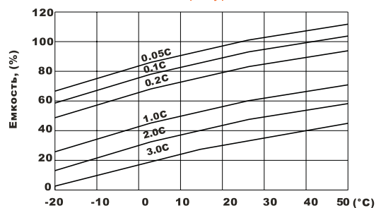
Влияние температуры на емкость
