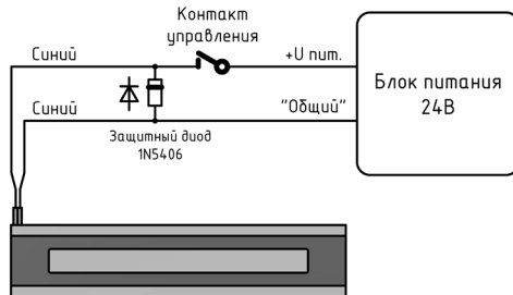
Рисунок 5 – Схема включения замка ALM-180FB-24V
