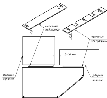
Рисунок 2 – Установка выравнивающих пластин под корпус и якорь
