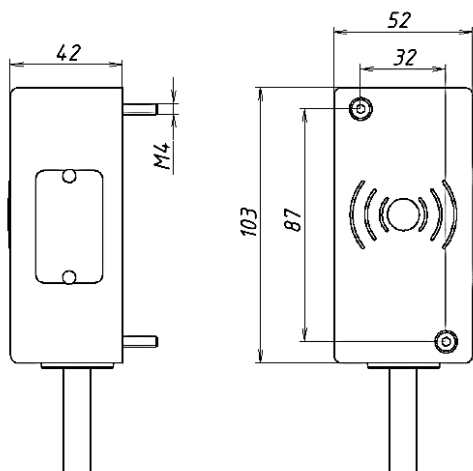
Рисунок 1 - Габаритно-установочные размеры считывателя ALM-PROX (вариант K)
