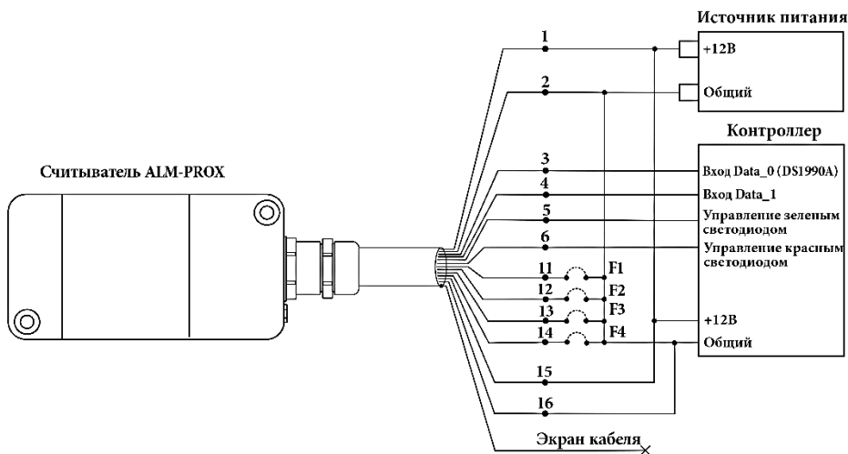
Рисунок 6 - Схема подключения считывателя ALM-PROX к контроллеру СКУД с питанием считывателя от одного источника питания.
