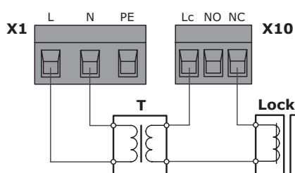
Рисунок 22. Схема подключения электромагнитного замка
