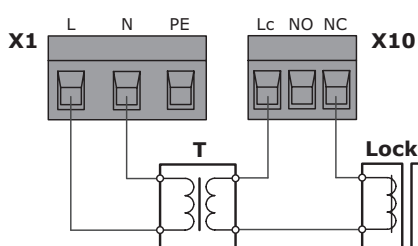
Малюнок 22. Схема підключення електромагнітного замка
